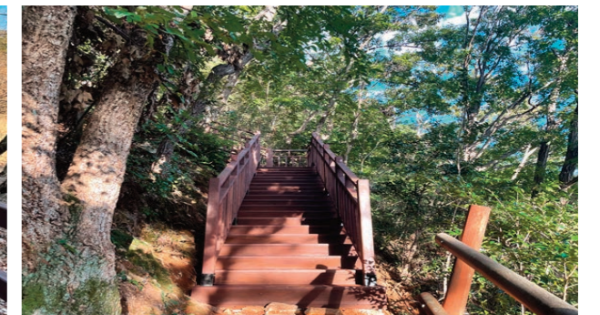
데크계단(신규)
